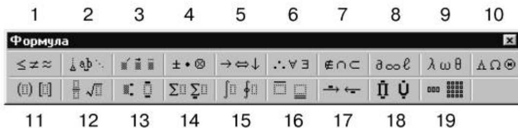
Рис. 3.1. Панель EquationEditor
